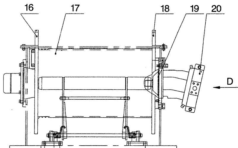
B向
