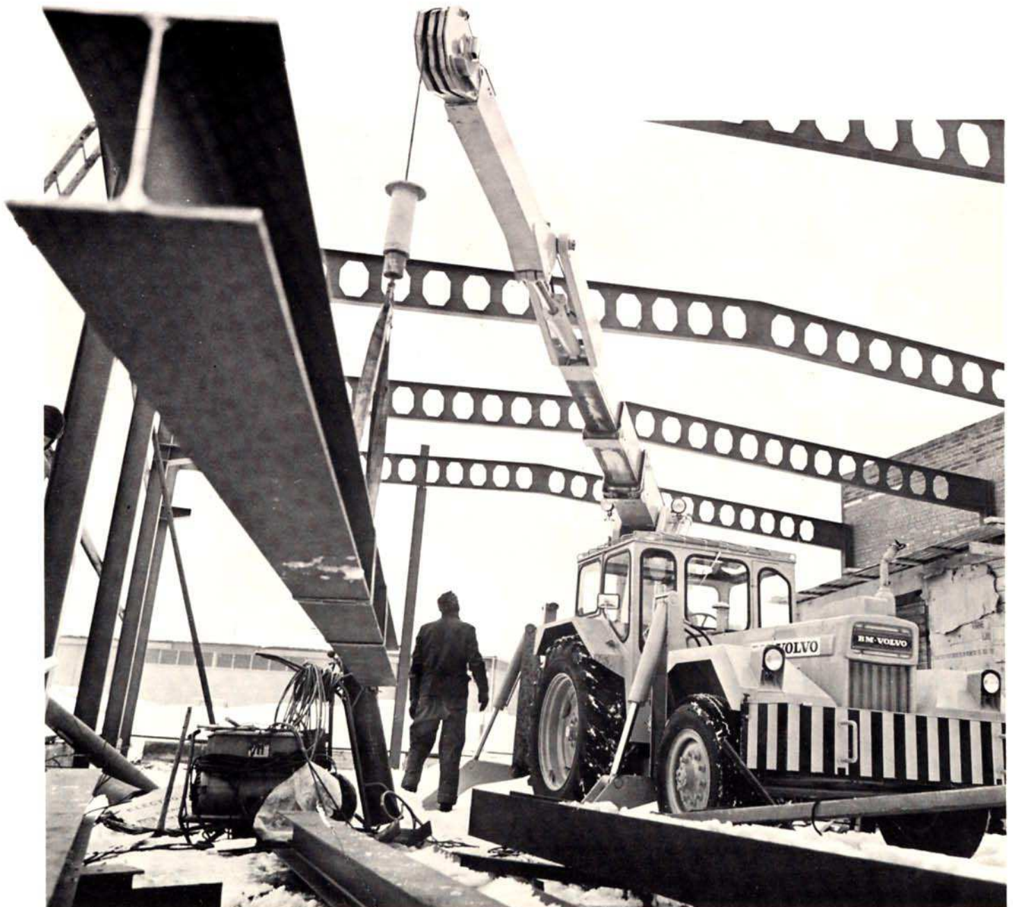
MK 691 kommer till sin rätt på trånga bygplatser. Maskinen kommer snabbt i arbetsposition och kranen arbetar följsamt och exakt med tung last. Räckvidd 11 m, Lyfthöjd 14 m.
