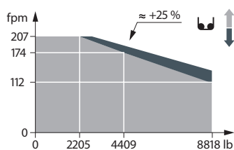
33 LVF 20 Optima
