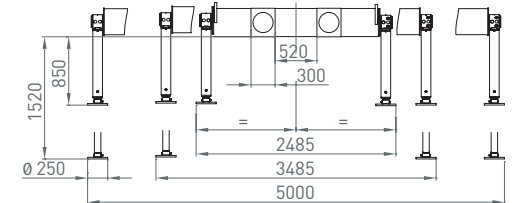
Vierkantabstützung squared outridge
