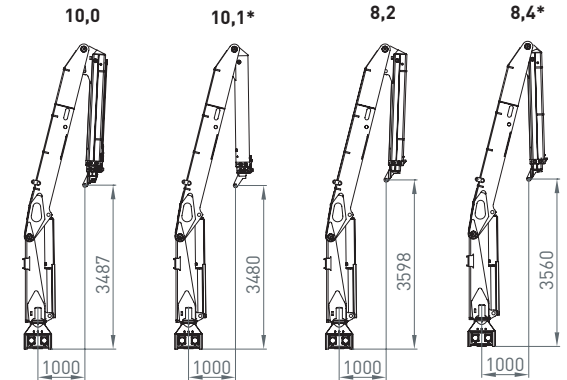
Schwenkabstützung swinging outridge
