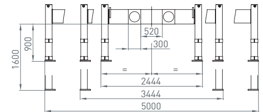
Vierkantabstützung squared outridge
