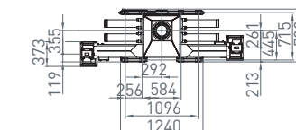
Seitensitz 02 universal rechts & links Side seat 02 universal right & left
