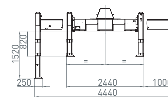
Vierkantabstützung squared outridge
