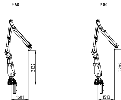
Sockel seitenverkehrt Crane base inverted
