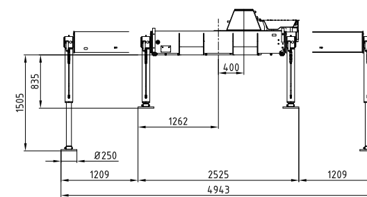
Sockel seitenverkehrt Crane base inverted
