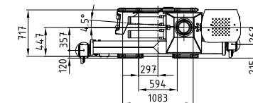
Seitensitz 02 universal rechts & links Side seat 02 universal right & left
