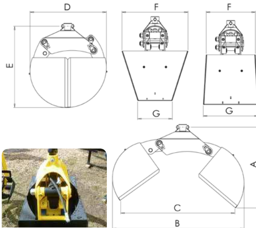
Łyżka dwuszczkowa dla rolnictwa montowana na chwytaku
