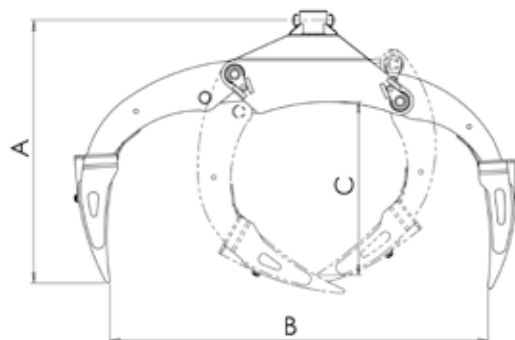
Łyżka dwuszczkowa do kruszywa montowana na chwytaku
