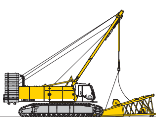
Entladung und Anbau des Auslegeranlenkstücks
