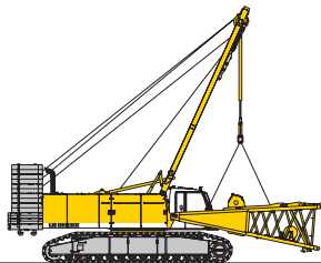
Entladung und Anbau des Auslegeranlenkstücks
