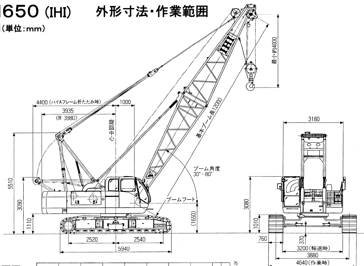
作業範圍圖
