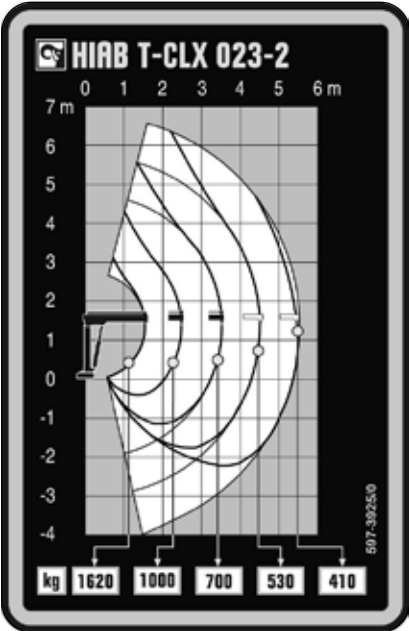
Load diagram HIAB T-CLX 023-2
