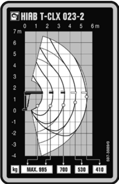
Load diagram HIAB T-CLX 023-2 CE
