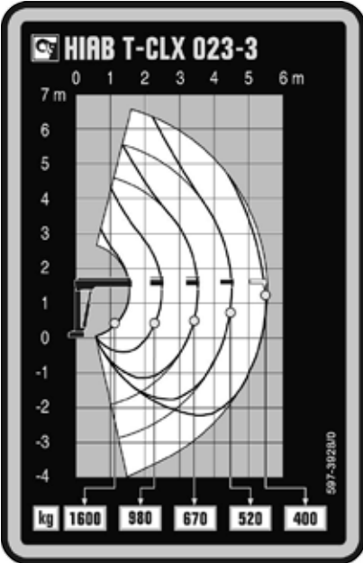
Load diagram HIAB T-CLX 023-3
