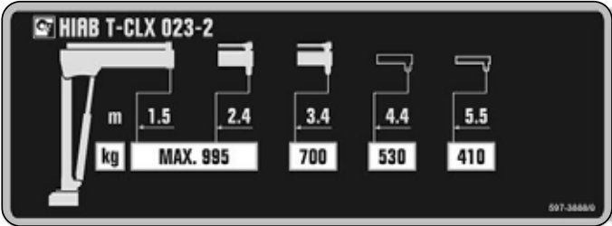
Capacity plate HIAB T-CLX 023-2 CE
