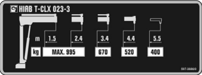
Capacity plate HIAB T-CLX 023-3 CE
