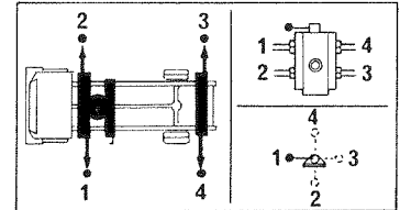
Schema di posizionamento del doppio comando
