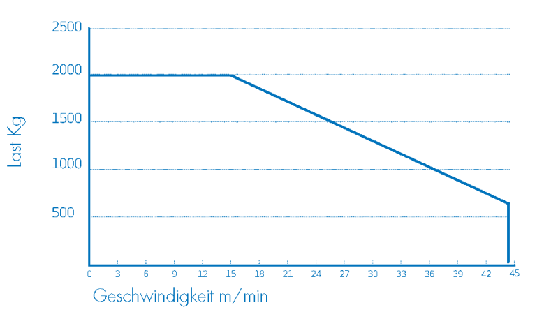
Hubgeschwindigkeit
