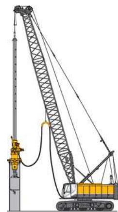
Flydrill
